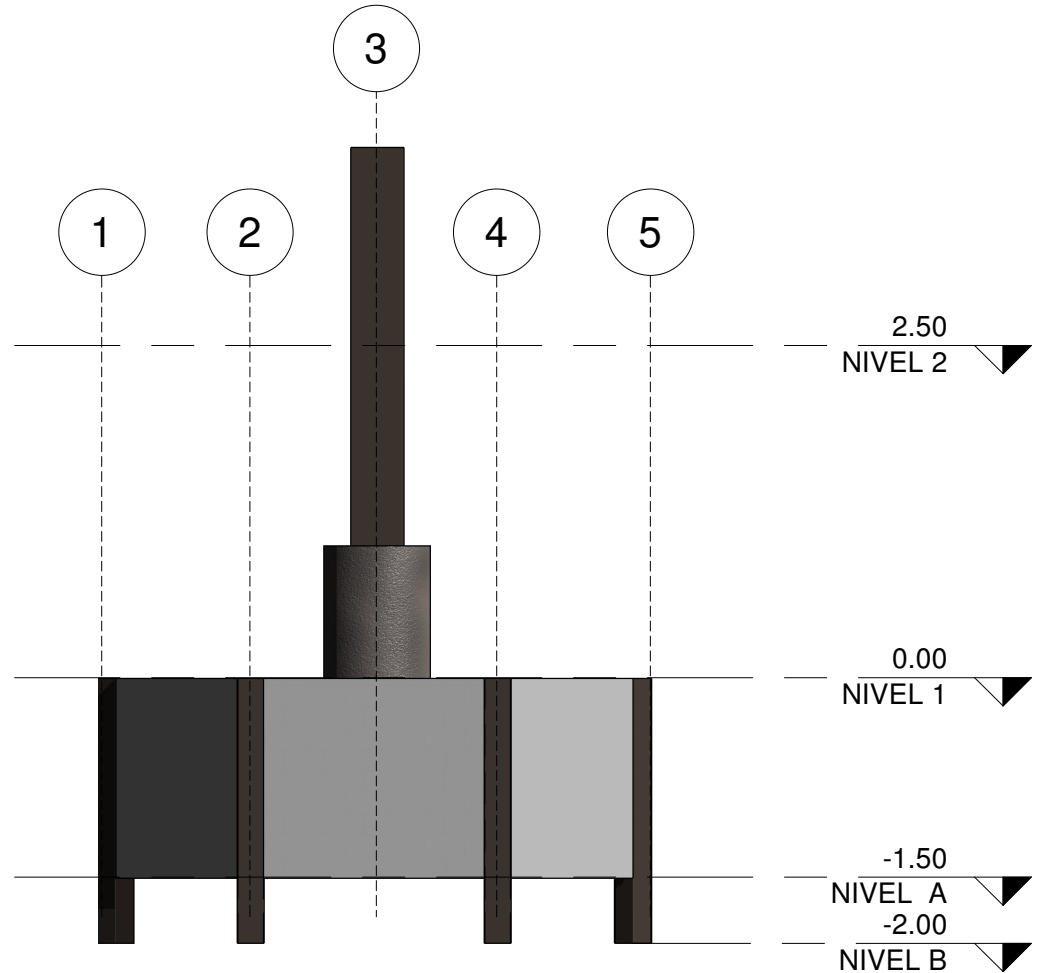
1 Vista Frontal 1 : 50
