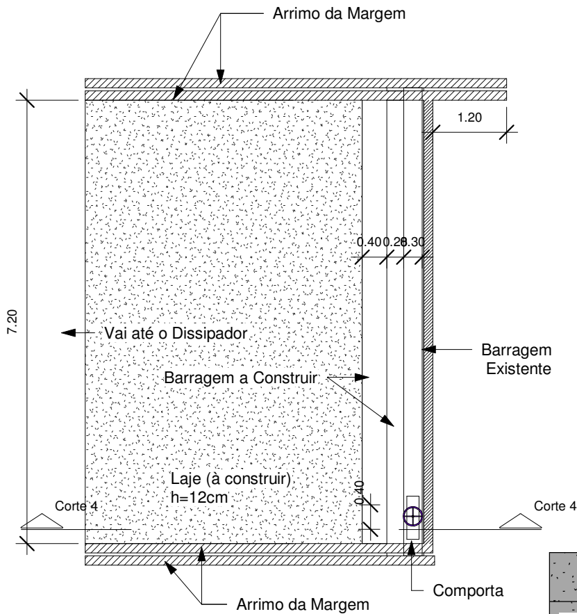
1 A1.1 Planta Barragem 1 : 75
