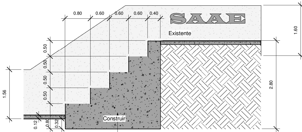
1 Corte 6 A1.5 1 : 50
