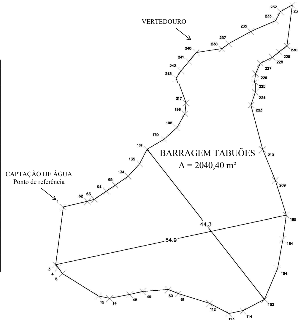
PLANTA BAIXA
