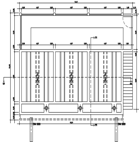
PLANTA BAIXA - FILTROS SOLDA LUB
