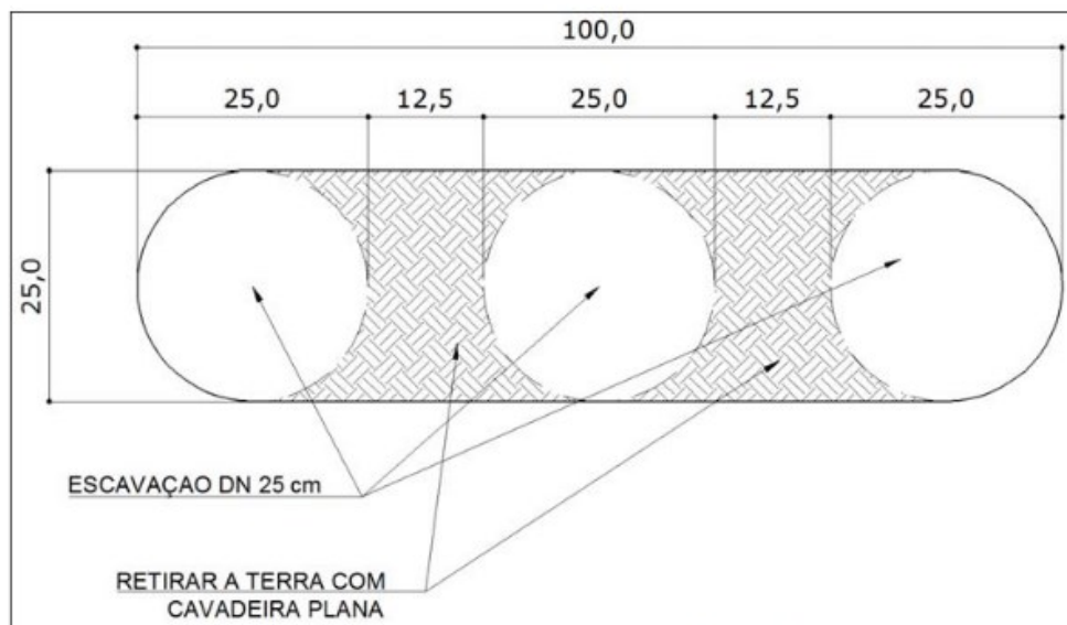
Figura 1 - Modelo de retângulo falsa-elipse
